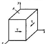
Рис. 3.3. Схема напряженного состояния в точке A
