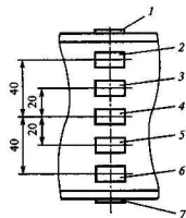
Рис. 3.5. Схема расположения тензорезисторов 1-7
