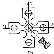
Рис. 1.20. Крестообразный плоский образец
