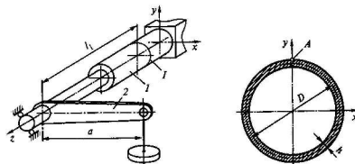
Рис. 3.1. Схема установки для испытаний на кручение:
