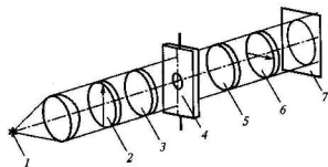
Рис. 3.57. Схема поляризископа
