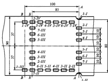
Рис. 3.46. Схема расположения тензорезисторов:
