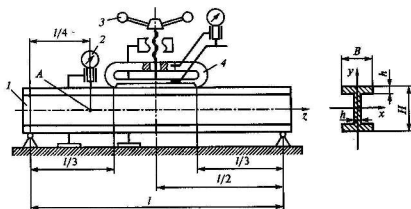
Рис. 3.4. Схема установки для испытаний на изгиб:
