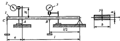
Рис. 3.15. Схема установки:
