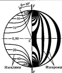
Рис. 3.60. Система изохром и изоклин
