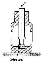
Рис. 1.10. Приспособление, применяемое при испытаниях на сжатие
