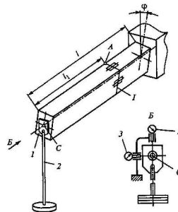
Рис. 3.8. Схема установки:
