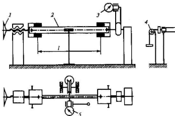
Рис. 3.54. Схема установки для изучения продольно-поперечного изгиба стержня:
