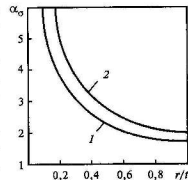
Рис. 3.49. Теоретические коэффициенты концентрации напряжений:
