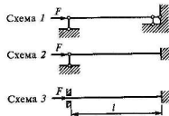
Рис. 3.51. Схемы закрепления стержня
