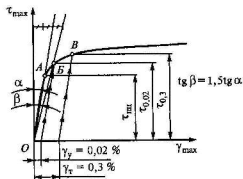
Рис. 2.15. Диаграмма сдвига материала
