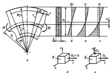
Рис. 3.34. Изгиб стержня в плоскости его кривизны
