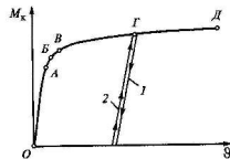
Рис. 2.11. Диаграмма кручения образца из пластичного материала:
