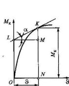
Рис. 2.14. Диаграмма кручения образца
