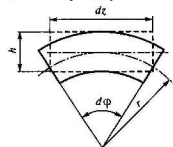
Рис. 2.23. Деформация элемента балки
