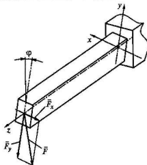
Рис. 3.13. Составляющие внешней силы F
