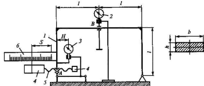
Рис. 3.29. Схема установки:
