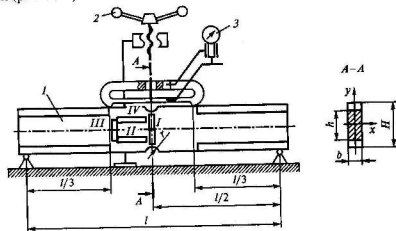
Рис. 3.45. Схема установки для изучения концентрации напряжений:
