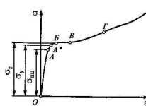
Рис. 1.15. Диаграмма сжатия низкоуглеродистой стали
