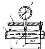
Рис. 2.21. Прогибомер:
