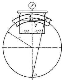
Рис. 2.22. Измерение кривизны балки
