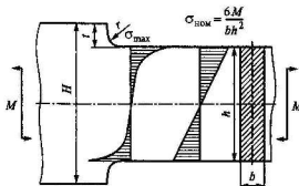
Рис. 3.48. Эпюры местных и номинальных напряжений
