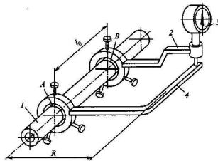
Рис. 2.25. Схема угломера:
