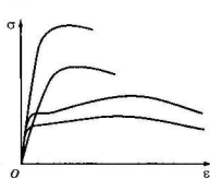
Рис. 1.7. Условные диаграммы растяжения материалов, находящихся в пластичном состоянии
