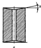
Рис. 1.13. Образцы с коническими торцами: a — с центральным отверстием; b — без отверстия
