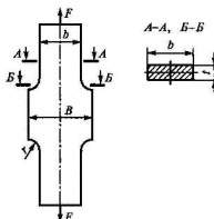
Рис. 3.61. Растянутая модель
