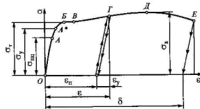
Рис. 2.4. Диаграмма растяжения низкоуглеродистой стали
