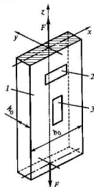
Рис. 2.17. Расположение тензорезисторов на стержне:
