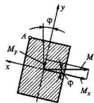
Рис. 3.11. Изгибающие моменты в сечении
