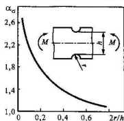
Рис. 3.47. Зависимость коэффициента концентрации напряжений от параметра 2r/h
