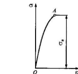
Рис. 1.16. Диаграмма сжатия серого чугуна
