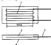
Рис. 2.18. Схема тензорезистора:
