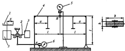
Рис. 3.25. Схема установки:
