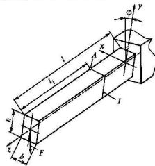
Рис. 3.10. Стержень
