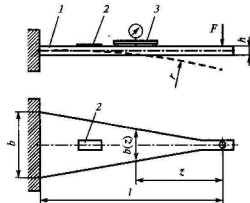
Рис. 2.20. Градуировочное приспособление:
