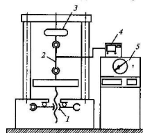
Рис. 2.16. Схема испытательной машины:
