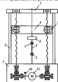
Рис. 2.1. Кинематическая схема испытательной машины:
