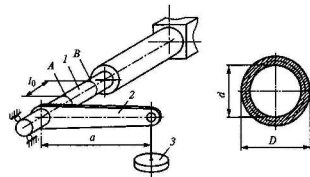
Рис. 2.24. Схема установки для испытаний на кручение:
