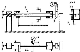
Рис. 3.50. Схема установки для изучения устойчивости стержня:
