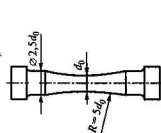
Рис. 1.4. Образец из хрупкого материала для испытаний на растяжение
