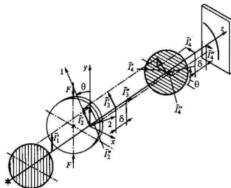
Рис. 3.59. Ход лучей в поляризископе
