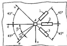
Рис. 3.37. Схема расположения тензорезисторов 1-3 в точке A сечения I
