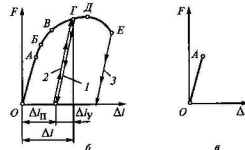
Рис. 2.3. Диаграммы растяжения образцов из низкоуглеродистой стали (а), конструкционной стали (б), серого чугуна (в)
