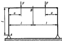
Рис. 3.27. Расчетная схема статически неопределимой плоской рамы
