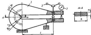
Рис. 3.32. Схема установки:
