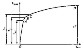
Рис. 1.18. Диаграмма сдвига металла, находящегося в пластичном состоянии
