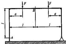
Рис. 3.26. Расчетная схема статически определимой плоской рамы
