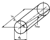
Рис. 2.12. Деформированное состояние расчетного участка образца при кручении
