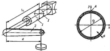
Рис. 3.36. Схема установки: 1 — стержень; 2 — рычаг
