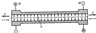
Рис. 1.19. Нагружение трубчатого образца
