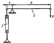
Рис. 3.58. Схема нагружения модели:
