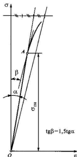
Рис. 2.5. Определение условного предела пропорциональности
